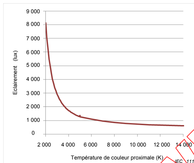
Figure 5 – Estimation du niveau d'éclairage énergétique où E_B = 1 \text{ W/m}^2 , frontière entre RG1 ( t_{\max} > 100 \text{ s} ) et RG2 ( t_{\max} < 100 \text{ s} ) en régime avec une petite source en fonction de CCT
