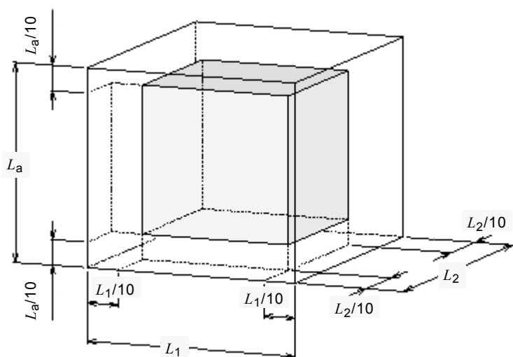
Figure 15 dans le cas d'une chambre rectangulaire ou cubique. Un espace approprié pour une chambre se situe dans l'intervalle excluant 1/10 de la distance entre les parois opposées comme le montre la
