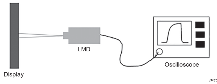
a) LMD plus oscilloscope
