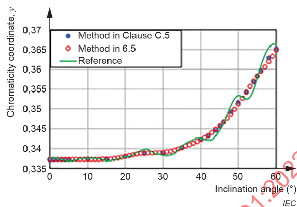
b) Chromaticity coordinate, y
