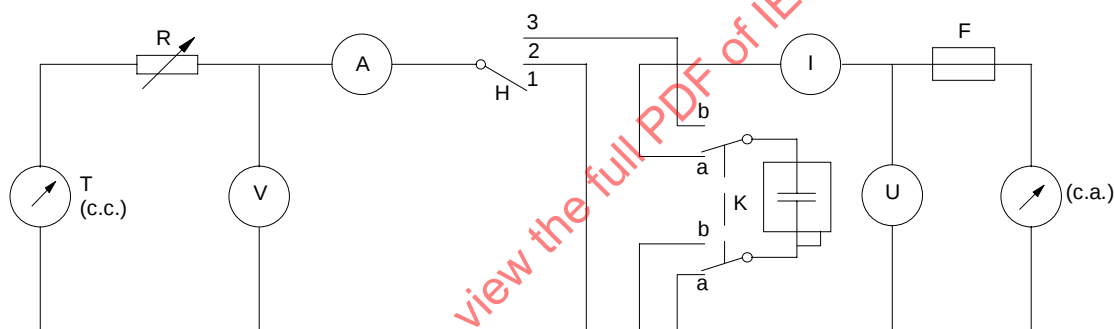
Figure 1 – Schéma pour effectuer l'essai de destruction
