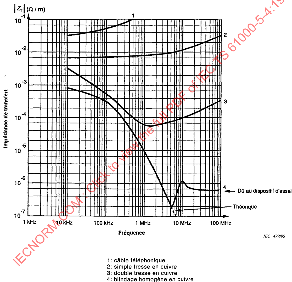
Figure 5 – Impédances de transfert expérimentales
