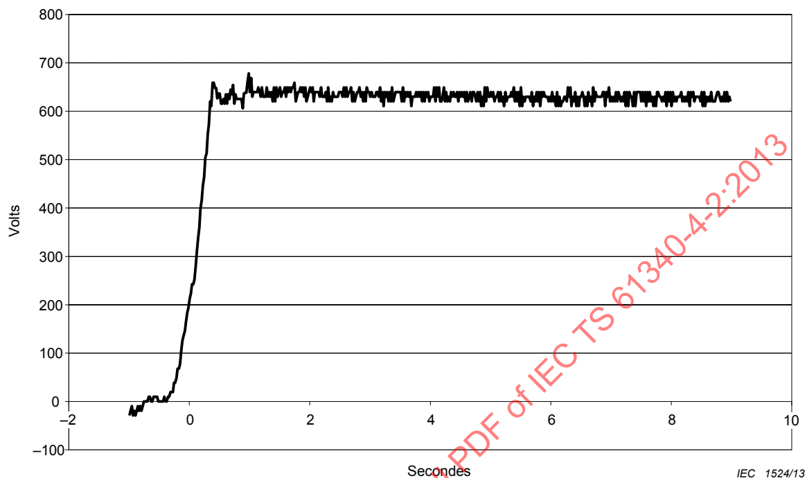
Figure B.2a – Tension de corps mesurée en se levant d'un siège en gardant les deux pieds ensemble
