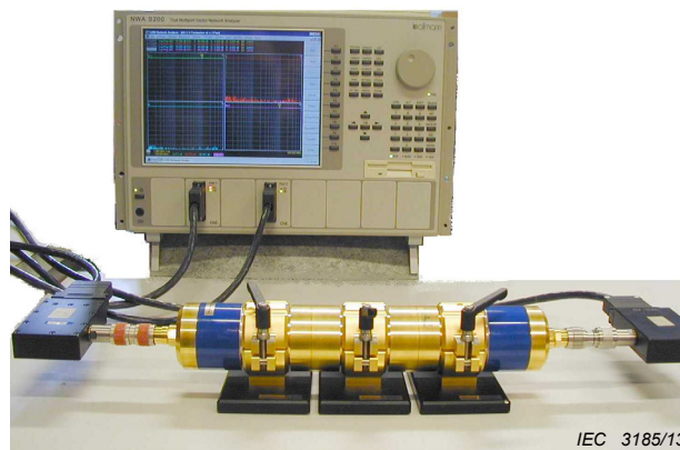
Figure 72 – S parameter test setup
