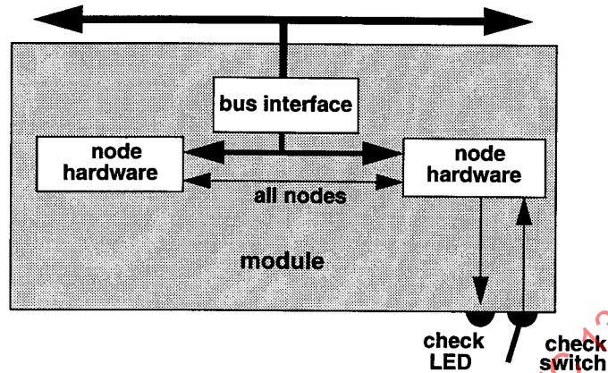
Figure 22—Multinode module
