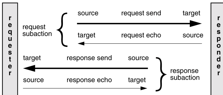
Figure 10 – Subactions
