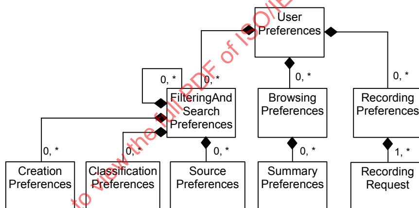
Figure 78 - The UserPreferences DS
