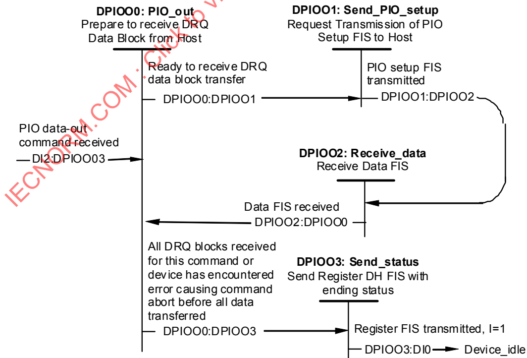
Figure 100 – PIO data-out command protocol (States DPIOO0-DPIOO3)
