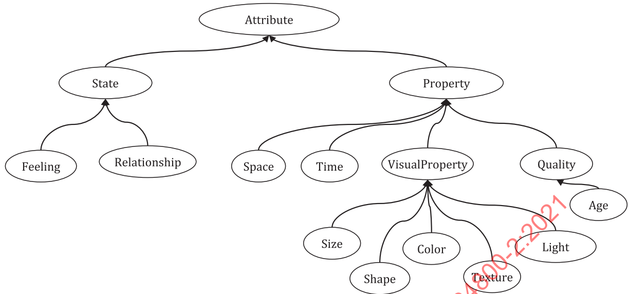
Figure 7 — Subclasses of jponeto:Attribute
