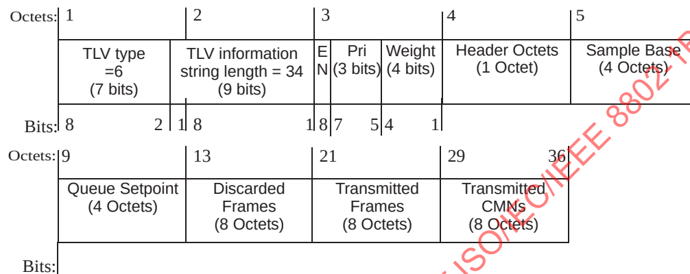
Figure 9-16—CN Parameters TLV
