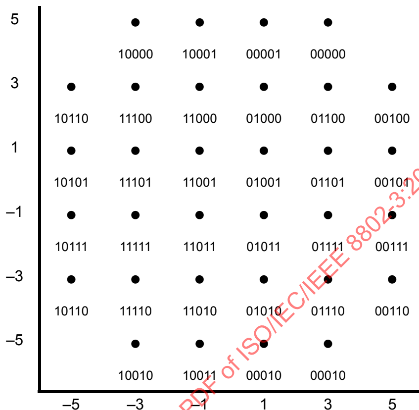
Figure 101-43—32-QAM
