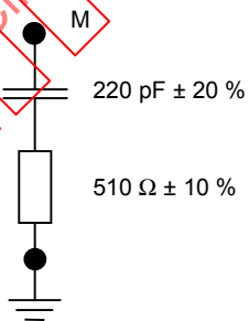
Figure 6 – Main artificielle, réseau RC (voir 6.2.5)
