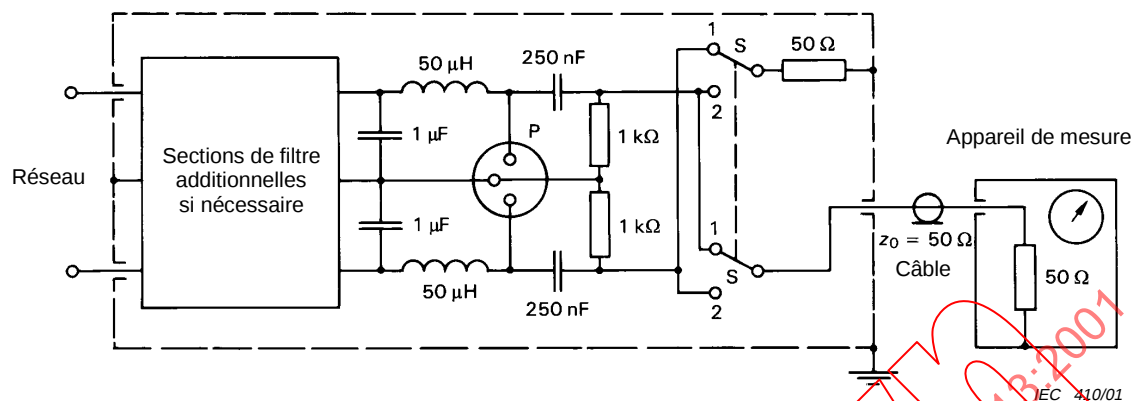
Figure 3 – Exemple d'un réseau fictif d'alimentation 50 Ω-50 μH (voir 5.3.1)
