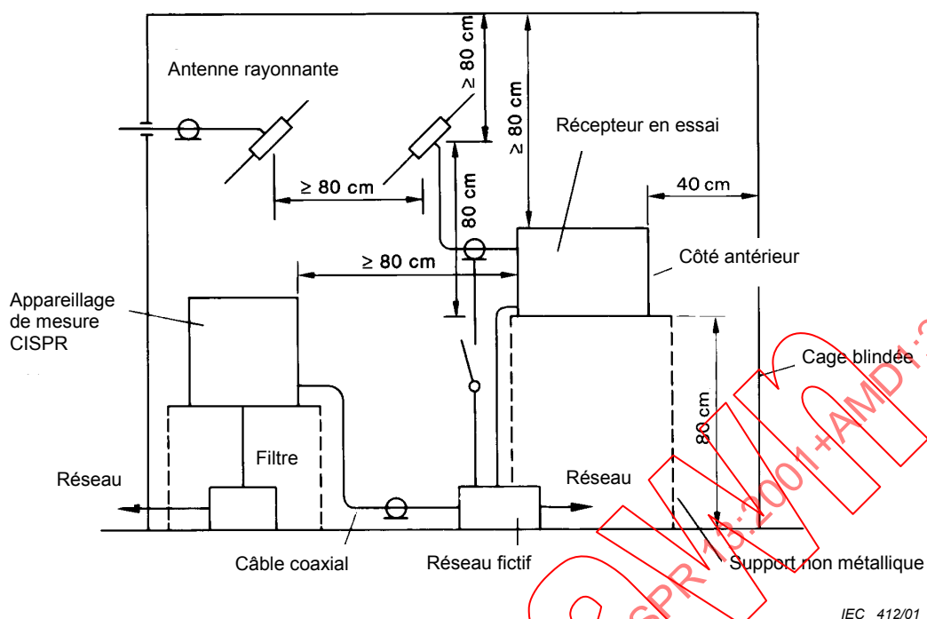
Figure 5 – Mesure de la tension perturbatrice à radiofréquence injectée dans le réseau (voir 5.3.1)
