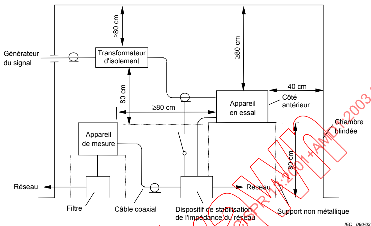
Figure A.1 – Mesure de la tension perturbatrice à radiofréquence injectée dans le réseau (voir 5.1.3 et 5.1.4) dans la gamme de fréquence de 150 kHz à 30 MHz (vue de côté)
