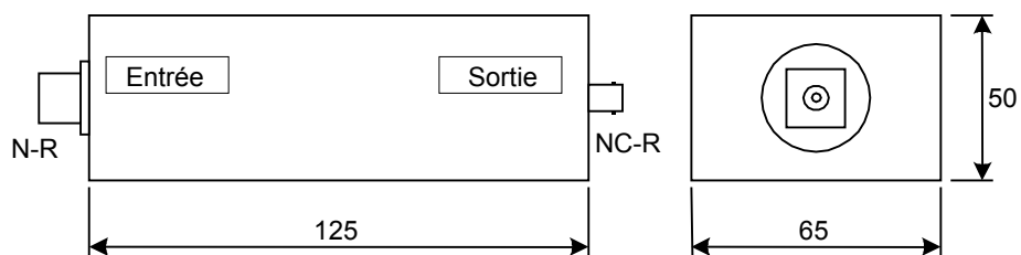
Figure A.3 – Dimensions typiques du transformateur d'isolement pour la gamme de fréquence de 46 MHz à 1,5 GHz
