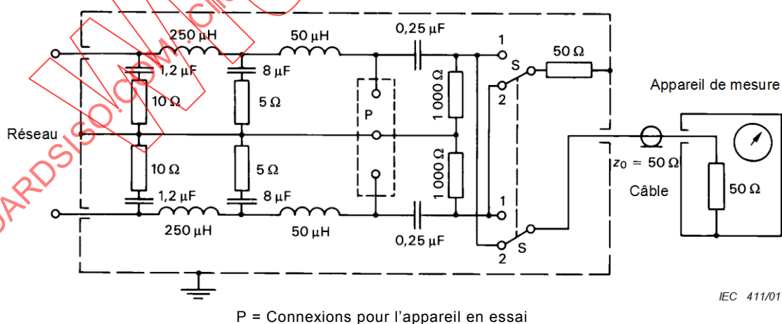
Figure 4 – Exemple de réseau fictif 50 Ω-50 μH-5 Ω (voir 5.3.1)
