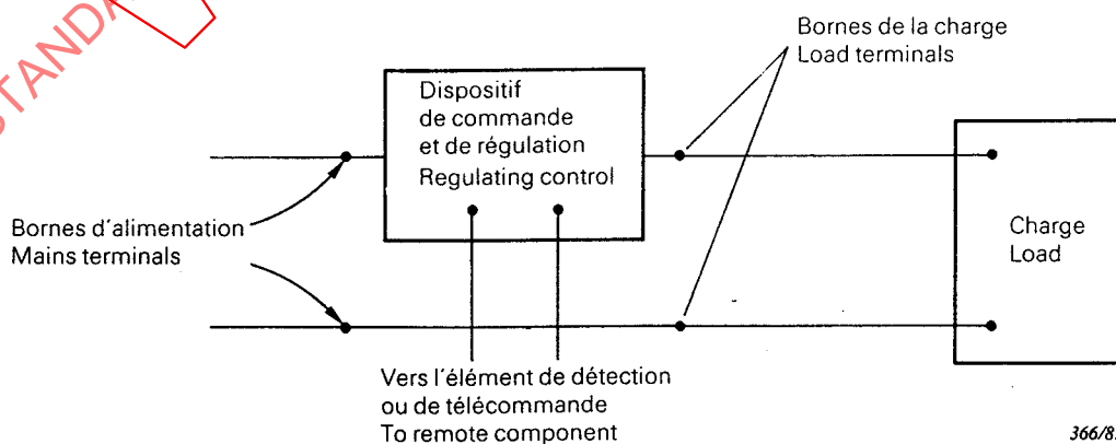
Figure 5a – Disposition dans le cas de la mesure d'un dispositif de commande et de régulation à deux bornes Measurement arrangement for two-terminal regulating controls
