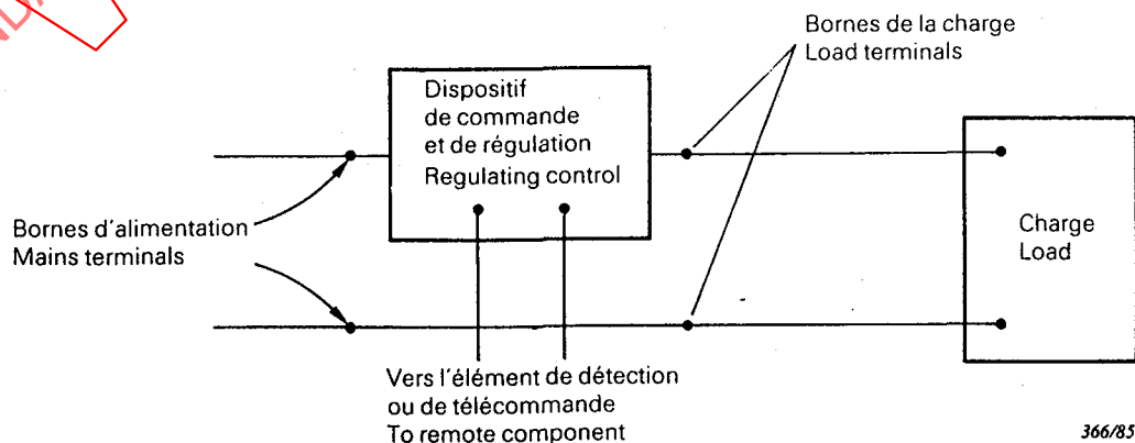
Figure 5a – Disposition dans le cas de la mesure d'un dispositif de commande et de régulation à deux bornes Measurement arrangement for two-terminal regulating controls
