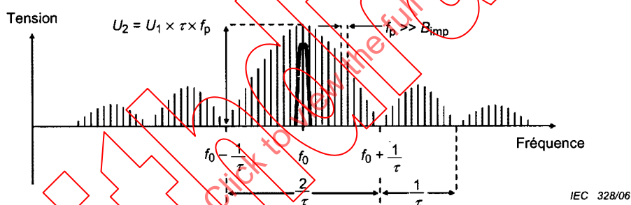
Figure E.5 – Filtrage avec une B_{imp} nettement inférieure à la prf
