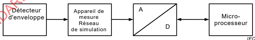
Figure 10 – Schéma fonctionnel d'un détecteur de valeur moyenne
