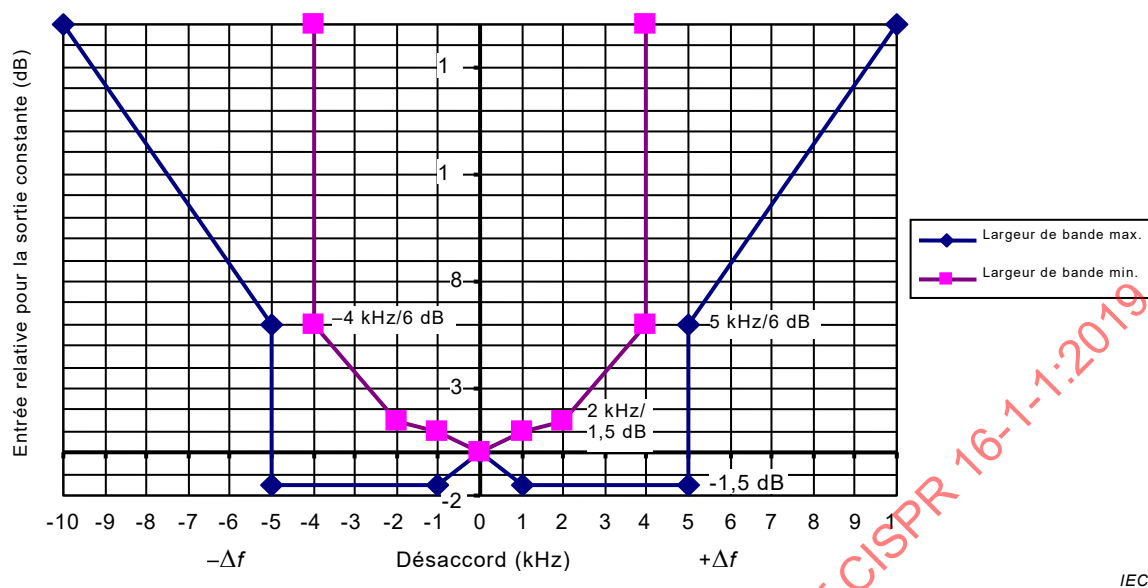
Figure 2 – Limites de la sélectivité globale – Bande passante (bande B)
