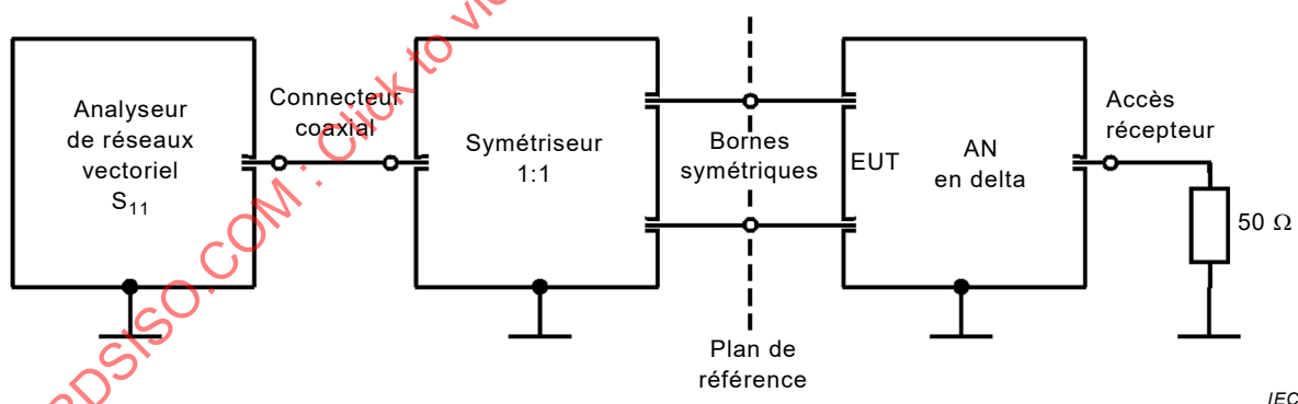
Figure K.2 – Montage de mesure de l'impédance symétrique
