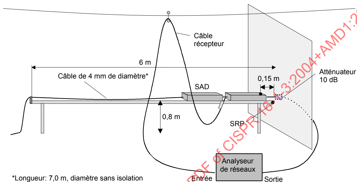
Figure C.1b – Montage pour les mesures de puissance sur l'ACTS ou l'ACRS
