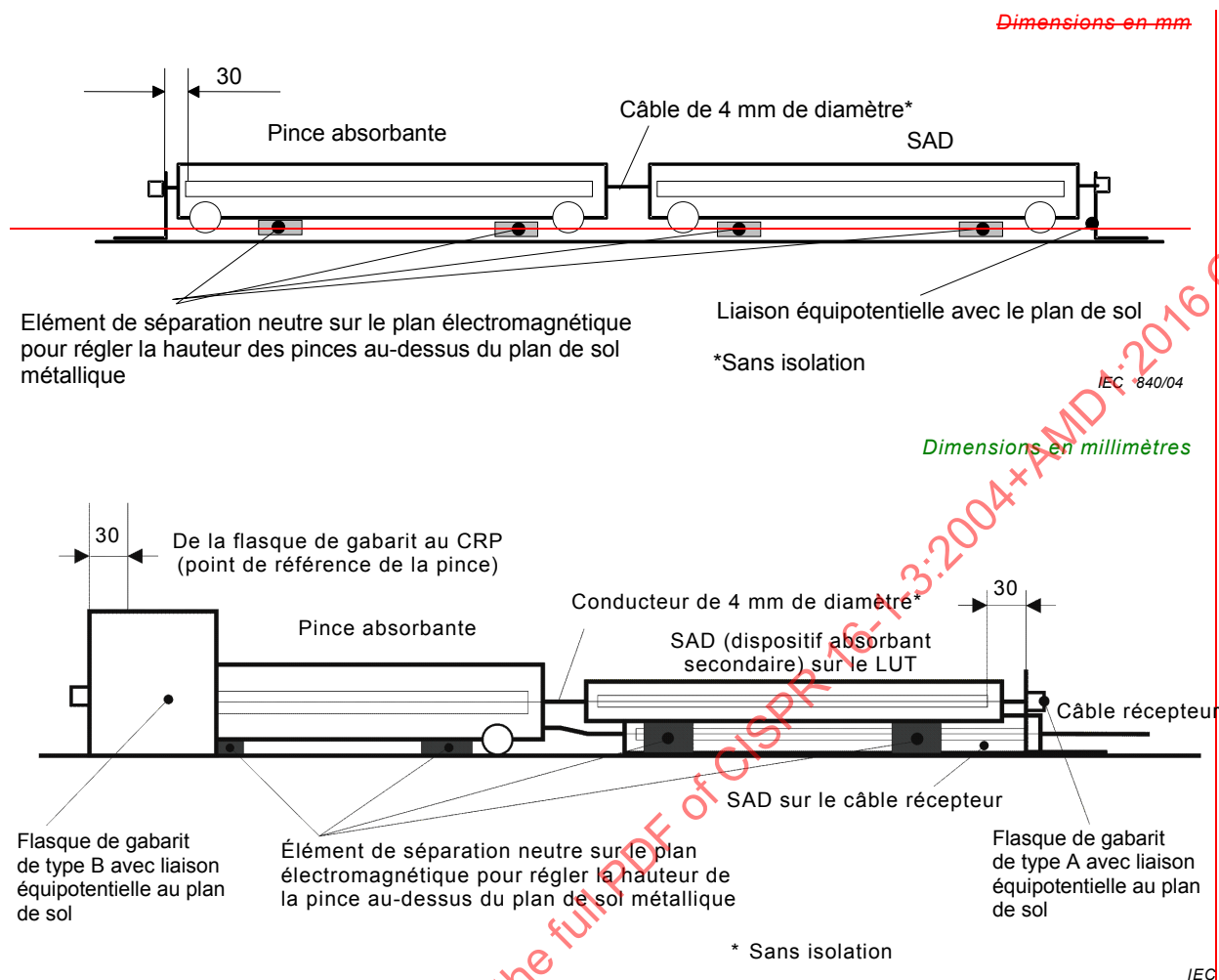
Figure B.3 – Vue latérale du gabarit d'étalonnage
