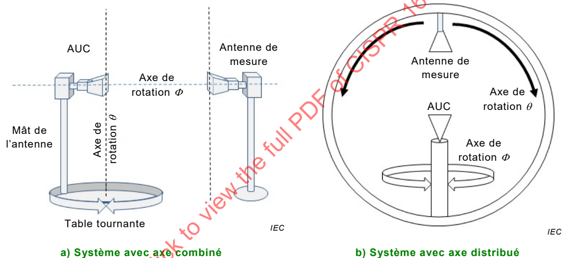
Figure I.1 – Montage d'essai classique pour le mesurage du diagramme de rayonnement d'une antenne
