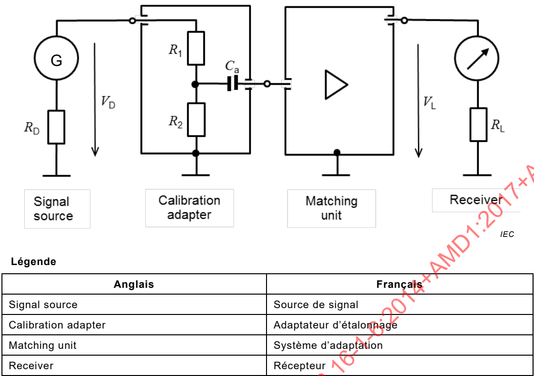
Figure G.10 – Circuit pour antenne fictive avec simulation des effets de la hauteur d'antenne effective h_e
