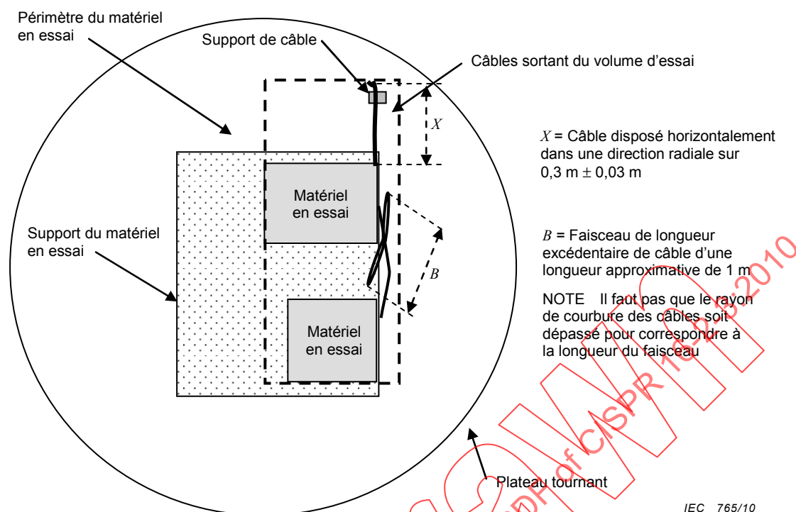
Figure 14 – Installation d'essai pour un matériel posé au sol, vue de dessus
