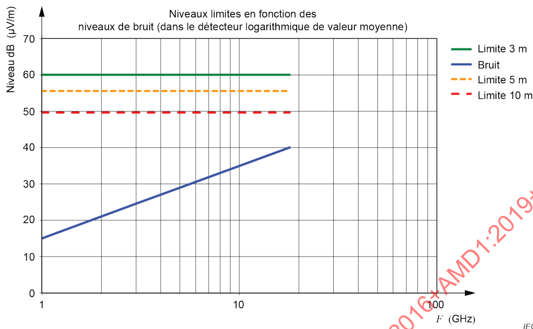
Figure F.8 – Niveau de bruit E_{\text{Nlogav}} (exemple pour 10\lg F_{\text{tot}} = 4 dB) comparé à la limite de perturbation E_{\text{Lav}} pour le détecteur logarithmique de valeur moyenne pour des distances de 3 m, 5 m et 10 m dans la plage de fréquences comprises entre 1 GHz et 18 GHz
