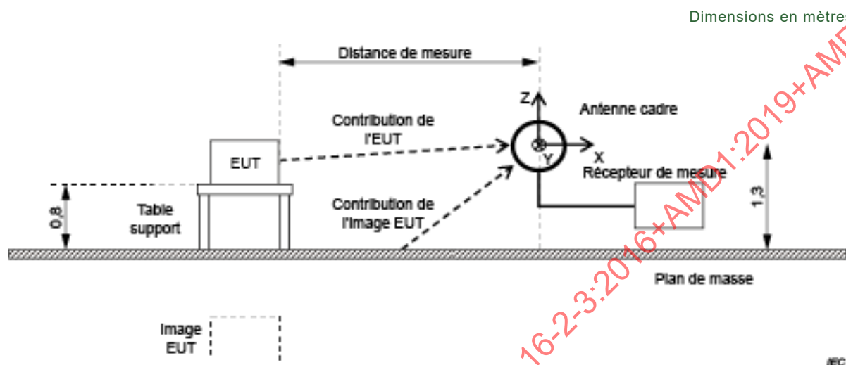
Figure 25 – Concept de l'installation pour les mesurages de l'amplitude de champ magnétique effectués à un emplacement d'essai en espace libre (OATS) ou dans une chambre semi-anéchoïque (SAC) pour l'EUT posé sur table
