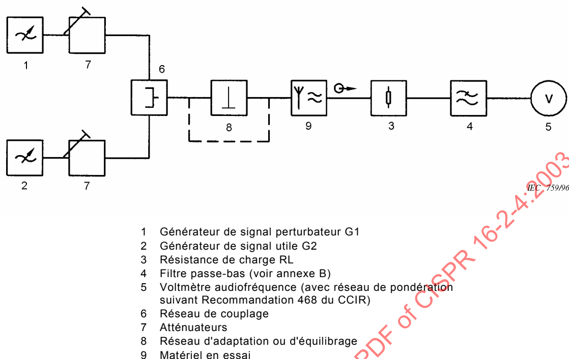
Figure 3 – Montage de mesure de l'immunité d'entrée des récepteurs de radiodiffusion sonore
