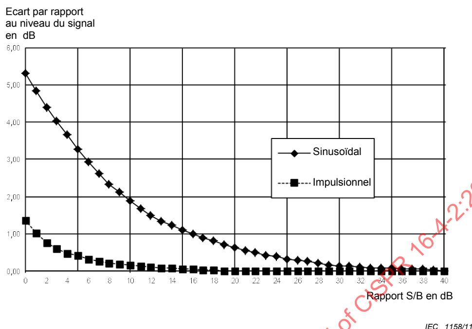
Figure A.1 – Écart de l'indication de niveau du détecteur de quasi-crête par rapport au niveau du signal à l'entrée du récepteur, pour deux cas: signal sinusoïdal et signal impulsionnel (PRF de 100 Hz)
