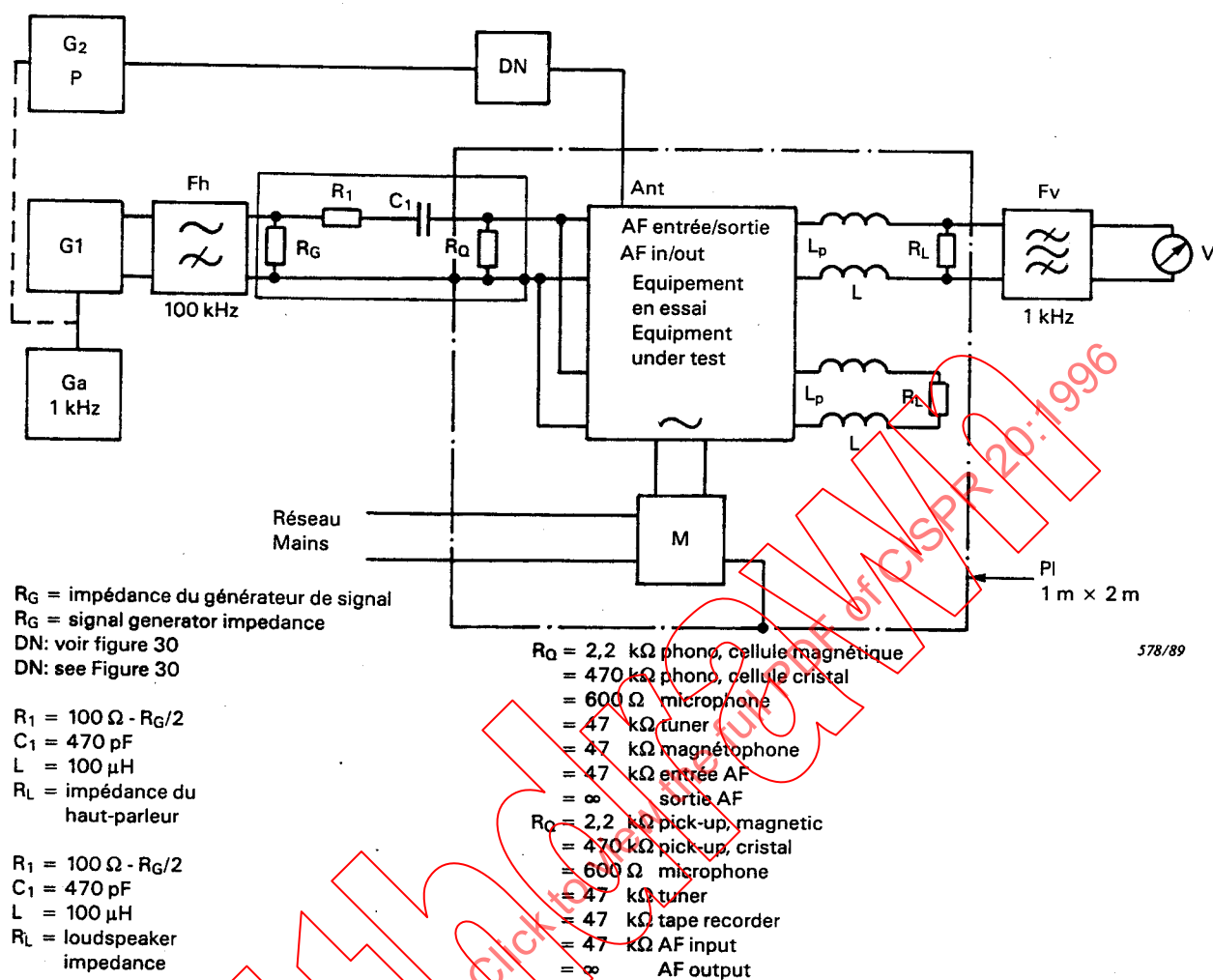
Figure 21 – Dispositif de mesure de l'essai d'immunité par la méthode d'injection de tension (bornes d'entrée/sortie audio (voir 5.5.2))
