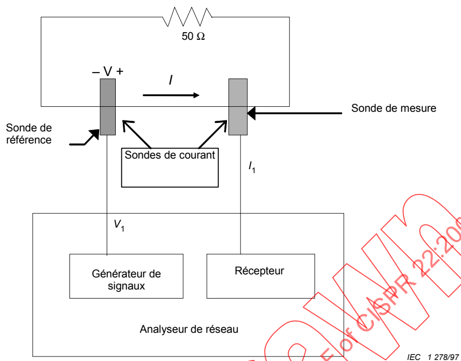
Figure C.4 – Dispositif d'étalonnage
