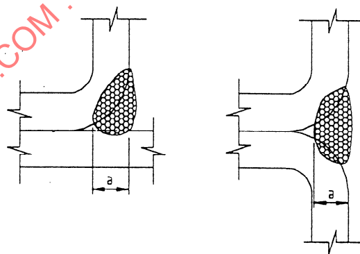
Fig. 8.9.7.11.a Flare grooves in RHS joints
