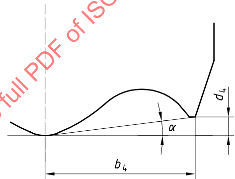
b) Concave bottom plus keel
