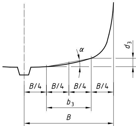
a) Straight bottom
