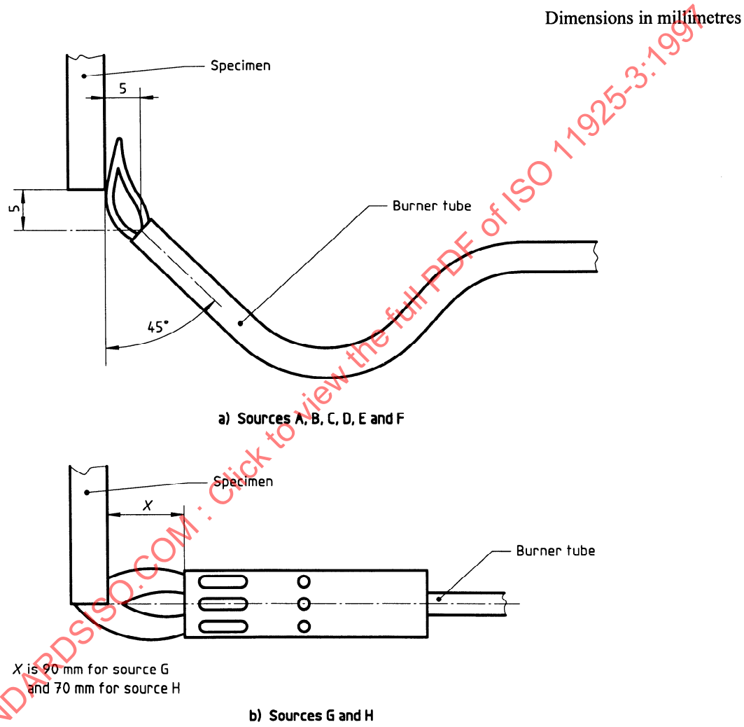
Figure 7 — Bottom edge ignition
