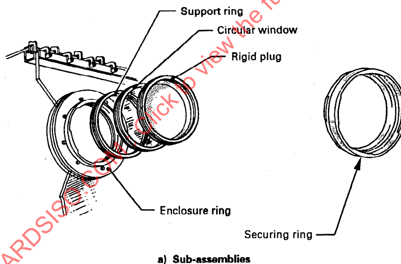
a) Sub-assemblies
