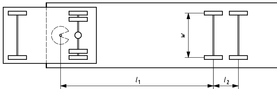
a) Semi trailer
