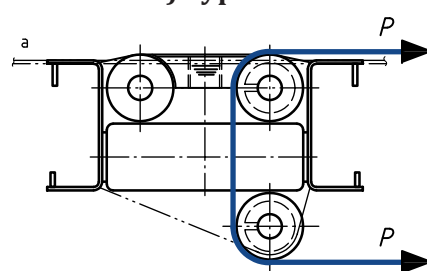
b) Type 4R
