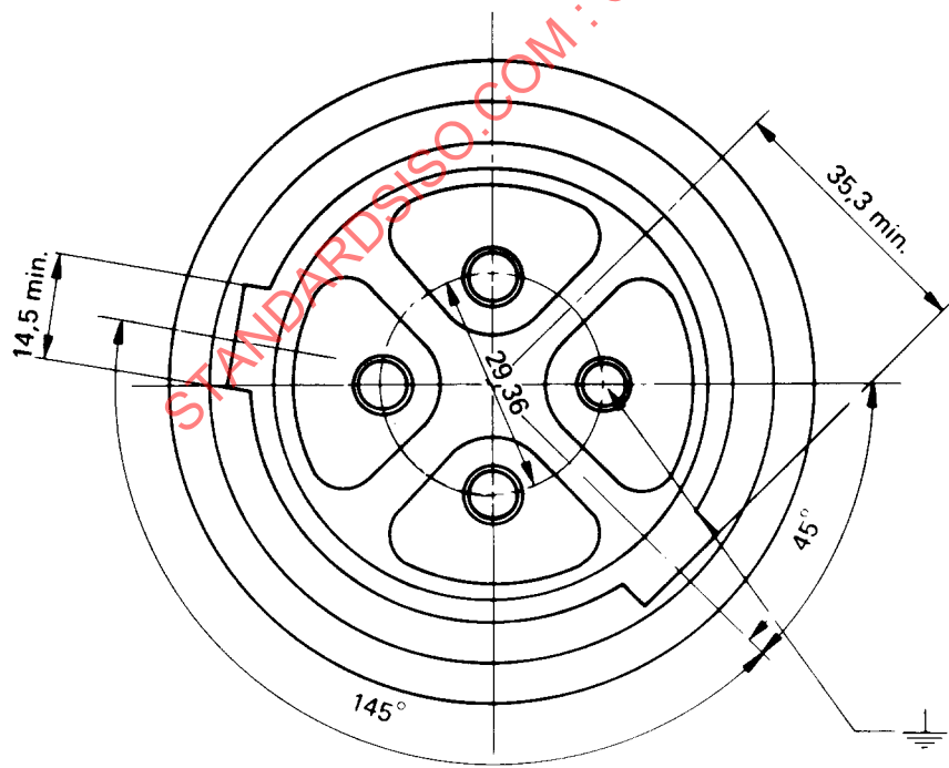
SOCKET
