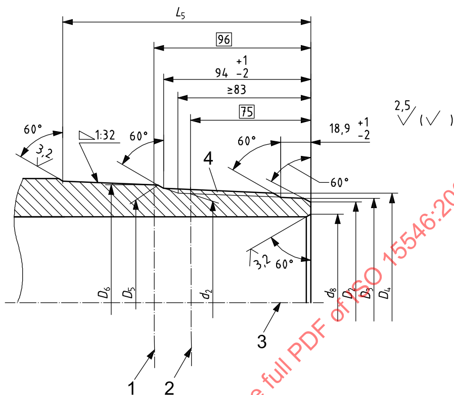
b) Drill pipe
