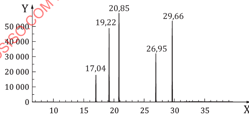
c) Chromatogram of a processed air sample. IS (DAIP): 17,04 min, DiBP: 19,22 min, DBP: 20,85 min, BBP: 26,95 min, DEHP: 29,66 min
