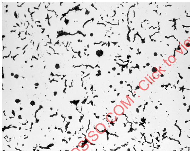
15 % nodularity
