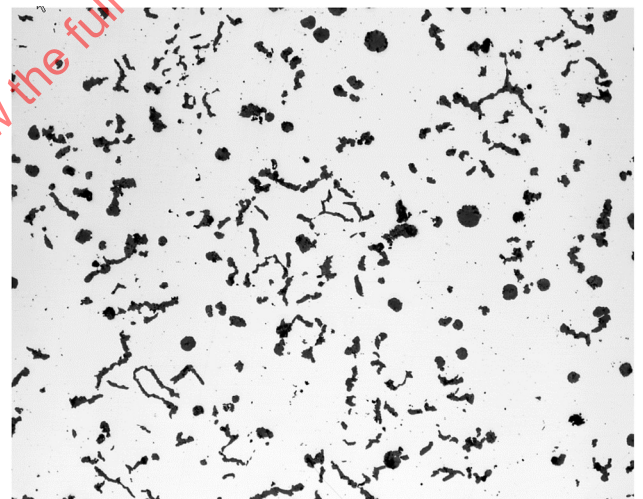
20 % nodularity
