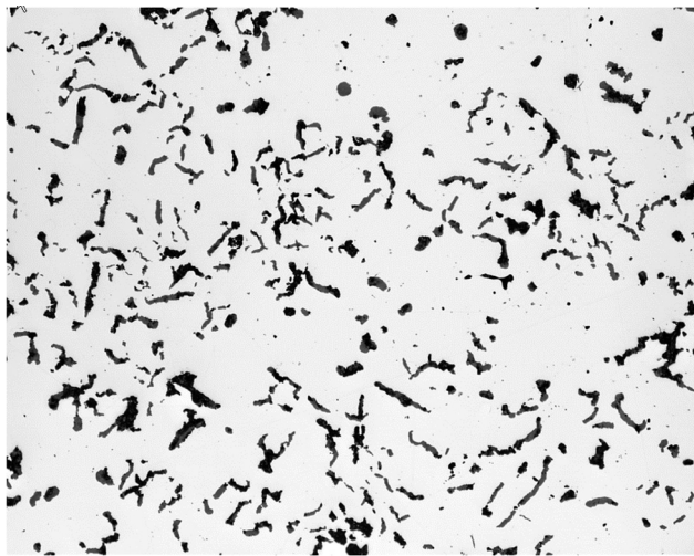
5 % nodularity
