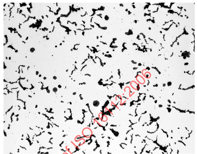
10 % nodularity
