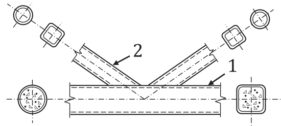
b) Gap K-joint
