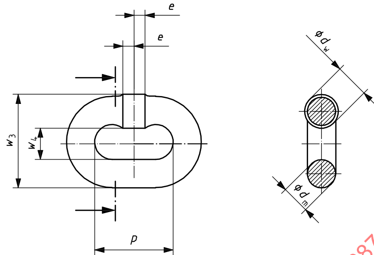
b) Type 1 — Link dimensions
