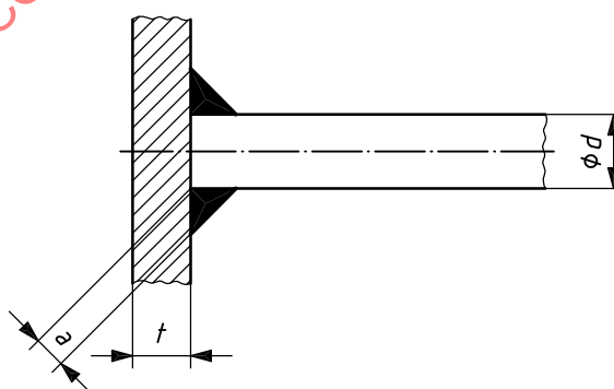
b) Set-in bar
