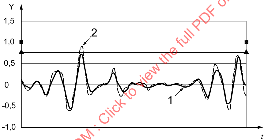
a) SDOF
