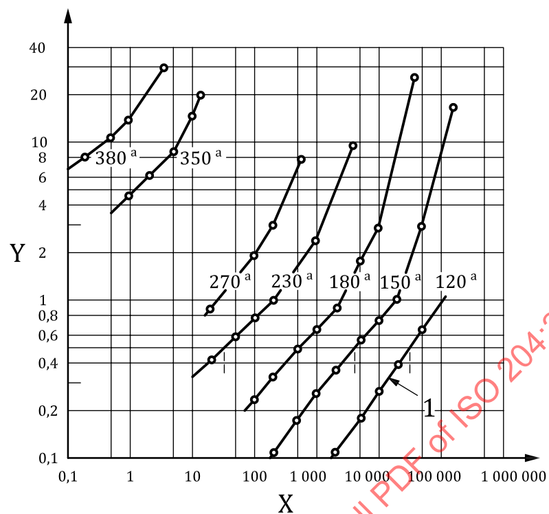
a) Creep diagram
