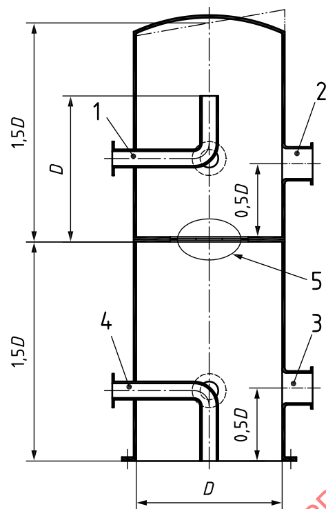
b) Test dome
