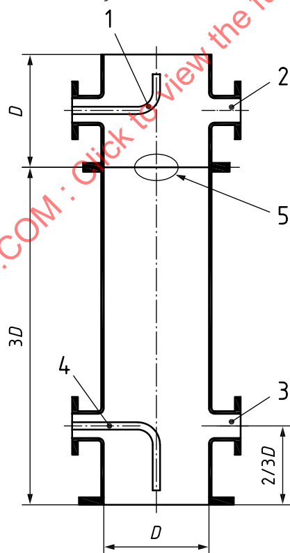
b) Test dome
