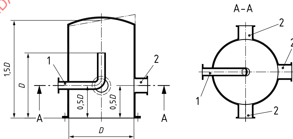
a) Test dome
