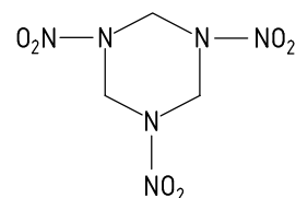
Hexogen (RDX)
