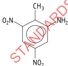
2-Amino-4,6-dinitrotoluene
