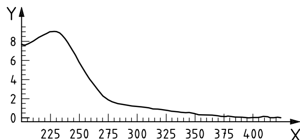
h) Tetryl
