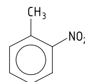
2-Nitrotoluene
