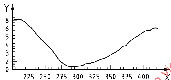
c) Hexyl
